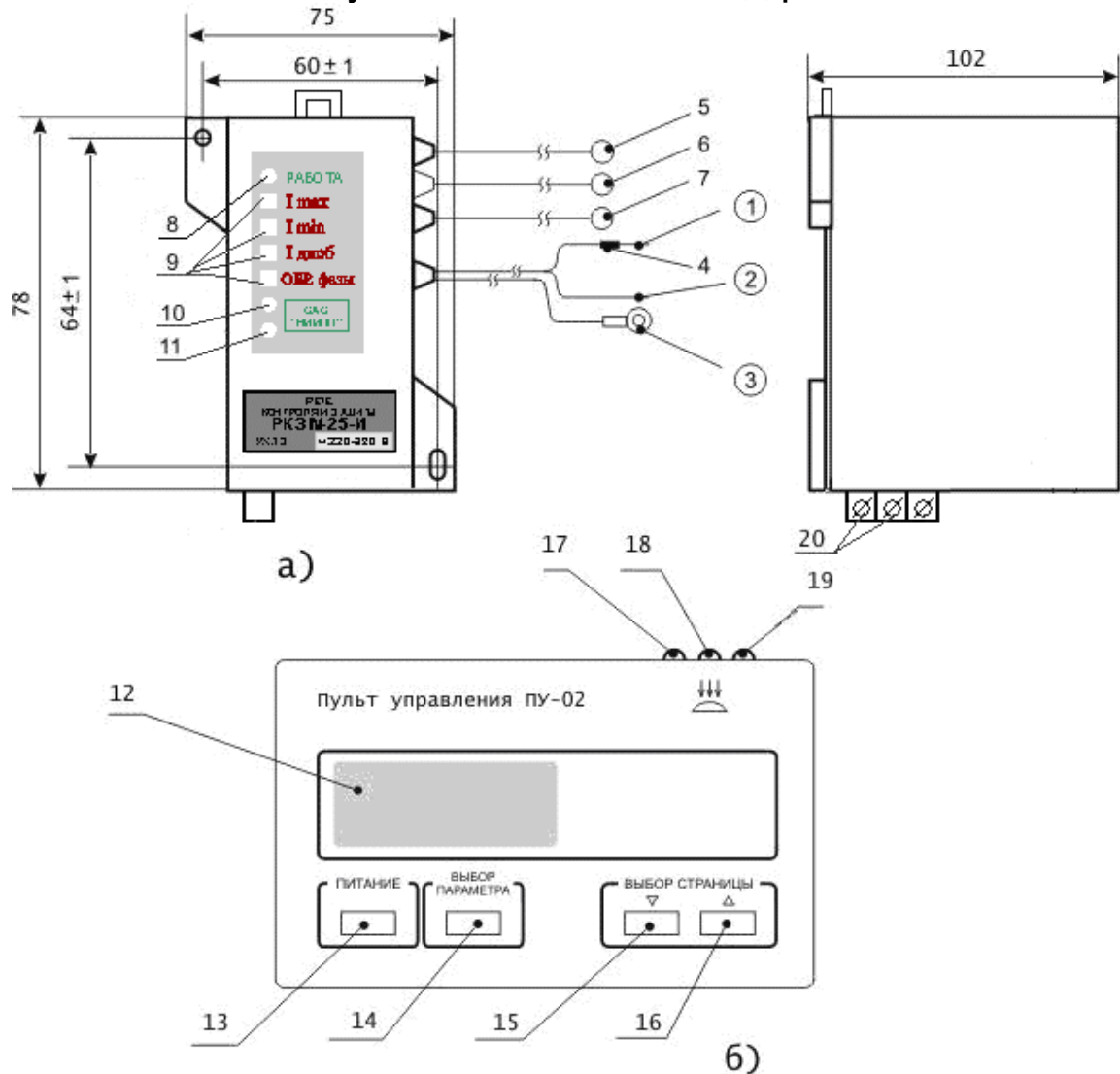
Рисунок 1 – Внешний вид реле
